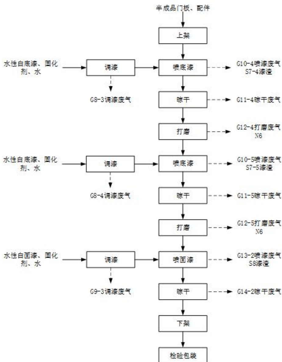
图 3-4 喷白漆工序生产工艺流程图
