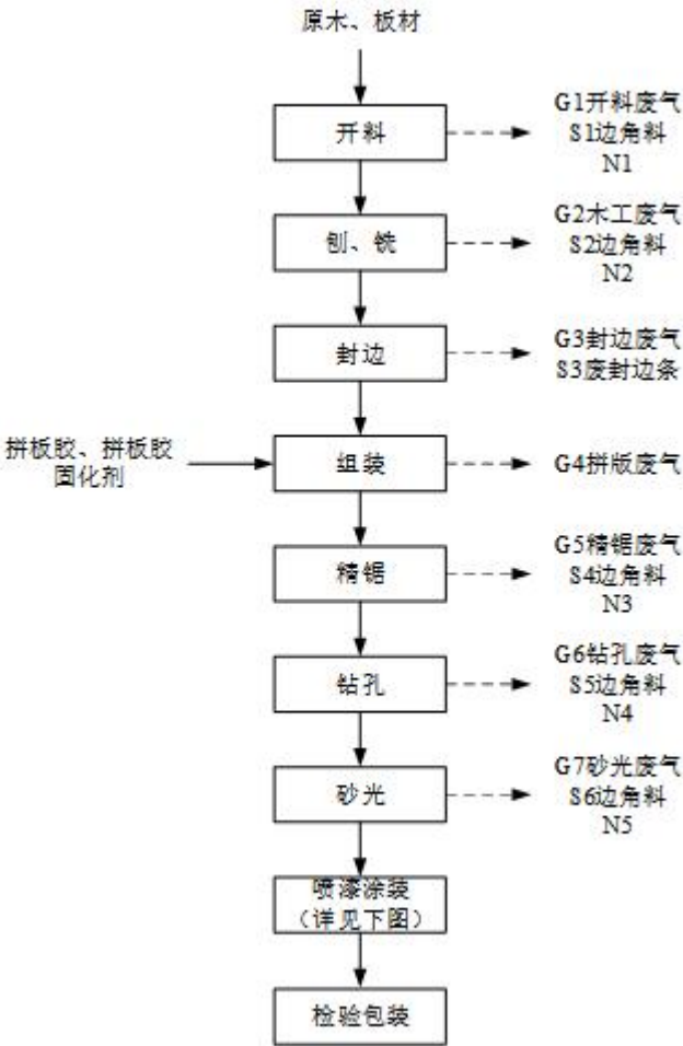
图 3-2 整体生产工艺流程图
