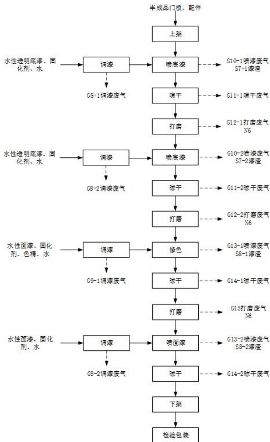
图 3-3 喷有色漆工序生产工艺流程图
