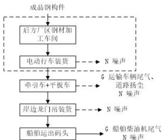
图 3-4 出港钢构件装卸工艺流程
