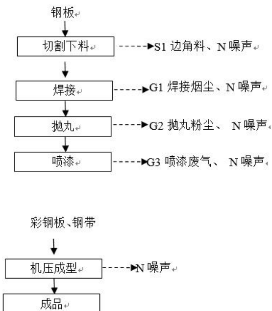
图 3-2 车间生产工艺流程图
