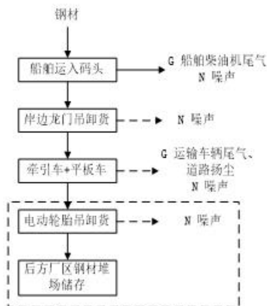
图 3-3 进港钢构件装卸工艺流程
