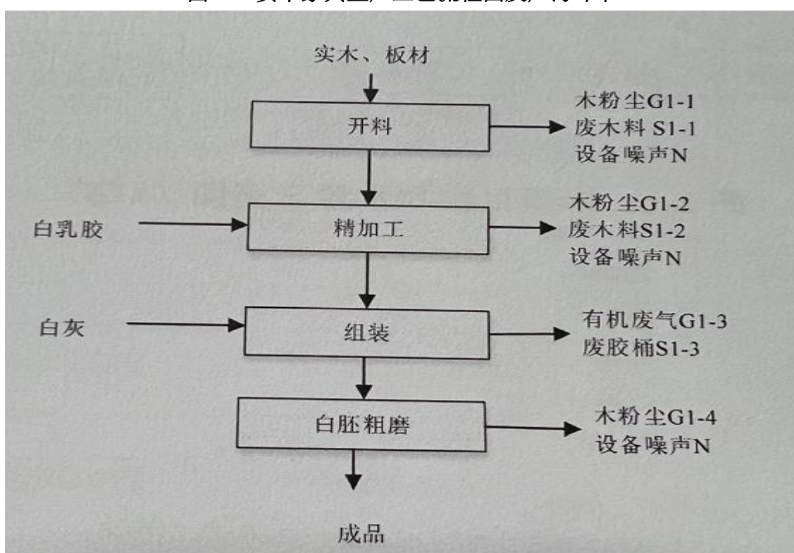
图 3-2 实木家具生产工艺流程图及产污环节
