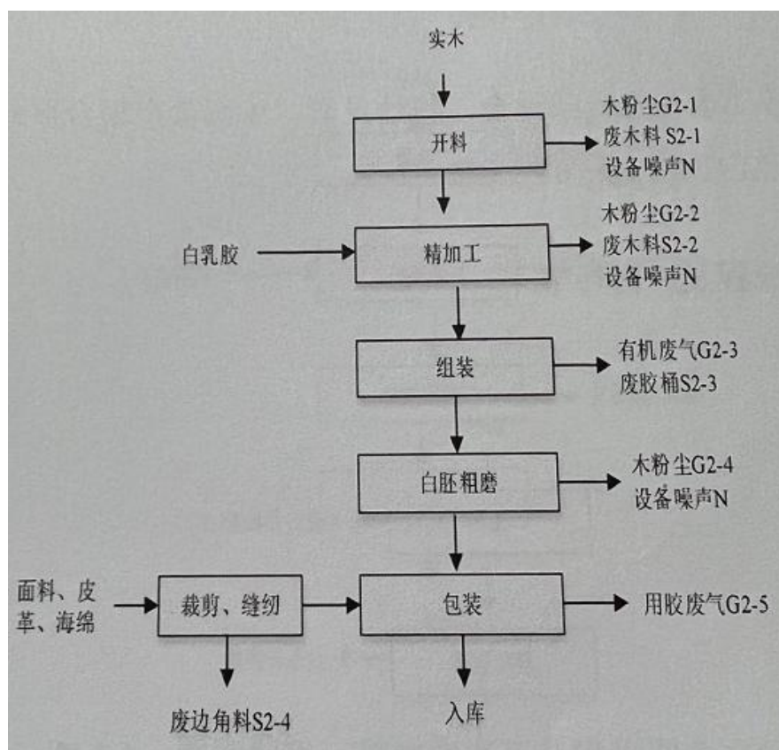
图 3-3 软包家具生产工艺流程图及产污环节
