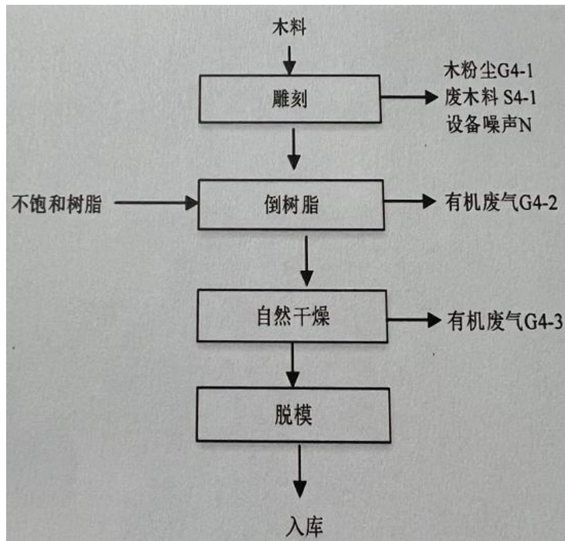
图 3-5 修饰图案、花纹生产工艺流程图及产污环节
